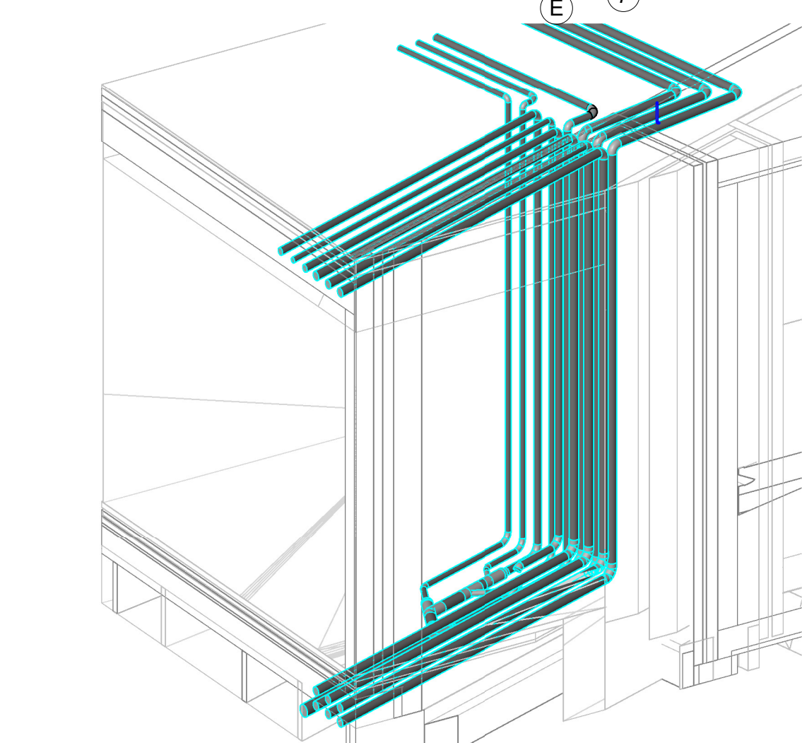
3 3D aanzichten standleidingen Pluvia
