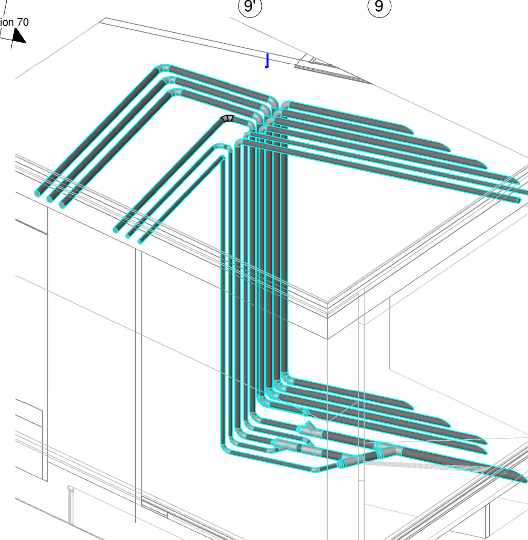
2 3D aanzichten standleidingen Pluvia
