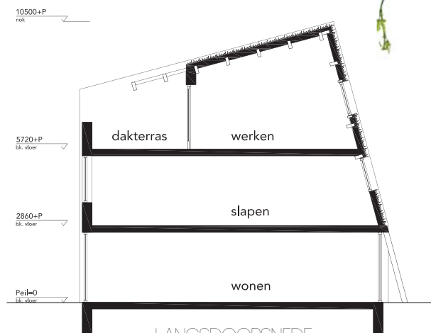
LANGSDOORSNEDE
