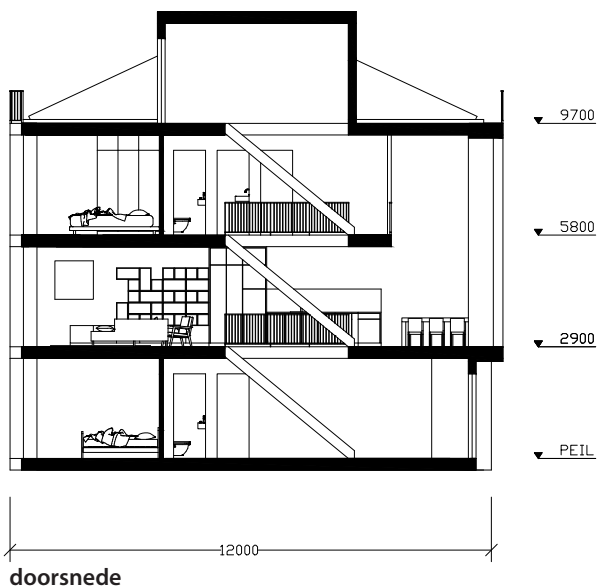
doorsnede
