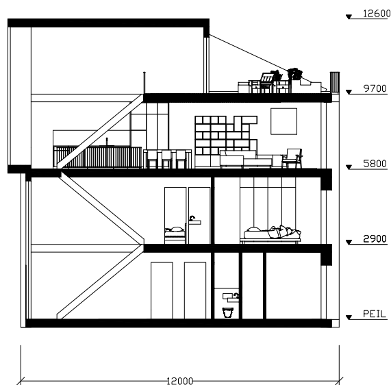
doorsnede
